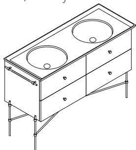
Umywalka podwójna L 130 / W 52 / H 88
