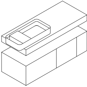
Umywalka z blatem L 128 / W 48 / H 71
