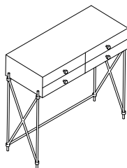
Toaletka L 80 / W 35 / H 74
