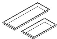
Półka L 37 - 56 / W 19 / H 4
